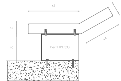
SECCIÓ E:1/20
