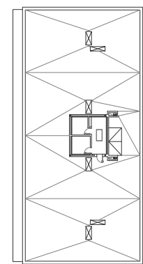
PLANTA SOTACOBERTA
