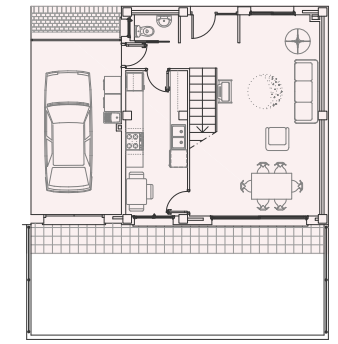
PLANTA BAIXA T1
